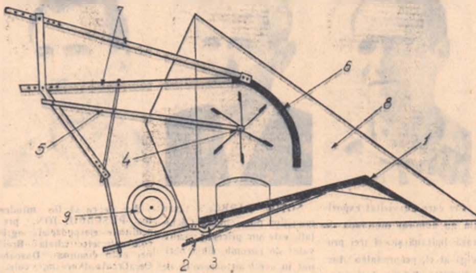
SCHEMA ADAPTĂRII COMBINĂI S. 4 PENTRU RECOLTAREA FLOREI-SOARELUI 1—ridicător, 2—suport fixare ridicător, 3—bara cu degete, 4—rabator, 5—console rabatorului, 6—aparatoare (scut), 7—consolele scutului, 8—aparatoare laterală, 9—melcul.
