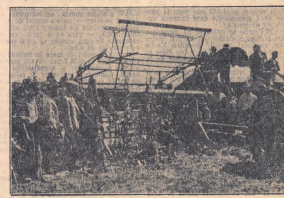
Combina sovietică S.K. 2,6 de recoltat și tocat porumb pentru siloz cu care a fost înzestrată nu de mult gospodăria de stat Agizea. Această mașină înlocuiește zilnic munca a 60 de oameni.
