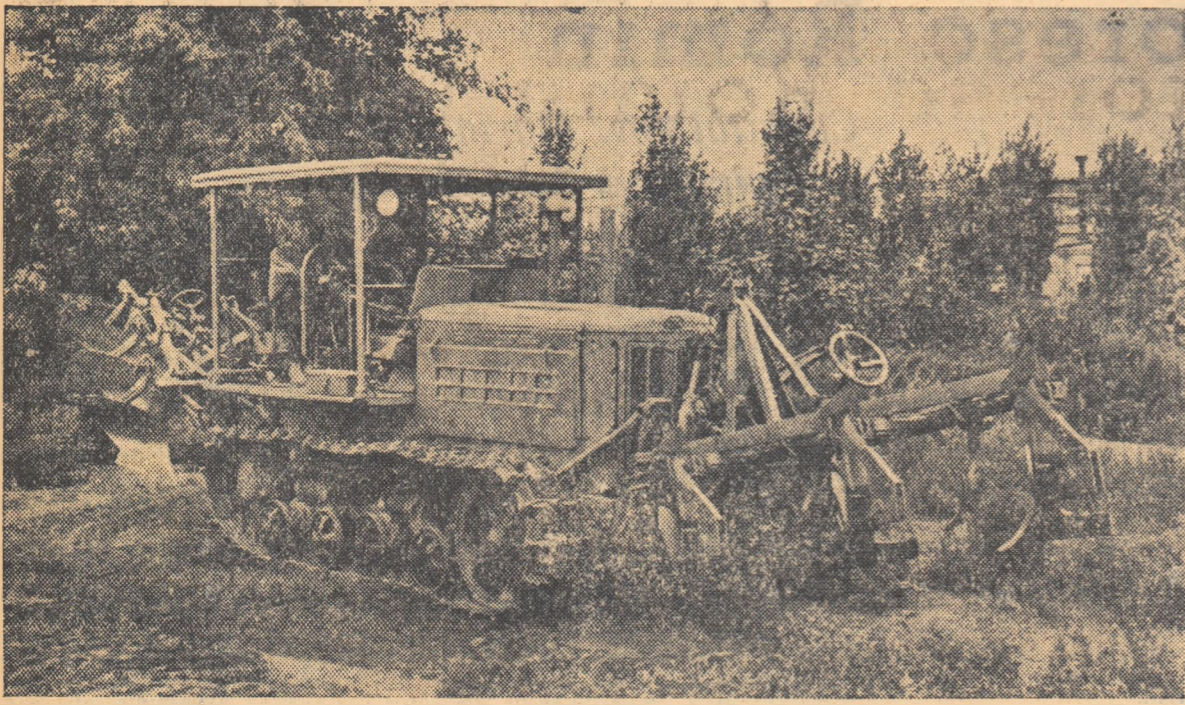
Uzina de tractoare din Stalingrad a fabricat un nou tip de tractor „D.T.-57 de pantă” destinat pentru lucrările de valorificare a terenurilor din regiunile muntoase ale țării. Acest tractor lucrează cu mașini suspendate așezate în fața și în spatele lui. În chișeu: noul tractor „D.T.-57 de pantă”.
