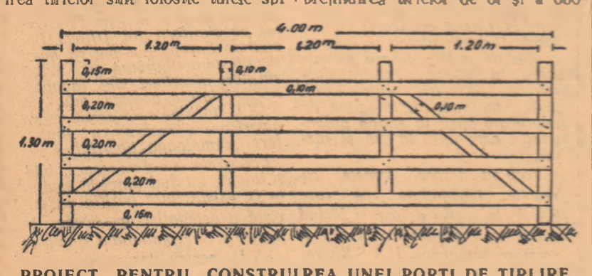
PROIECT PENTRU CONSTRUIREA UNEI PORȚI DE ȚIRLIRE
