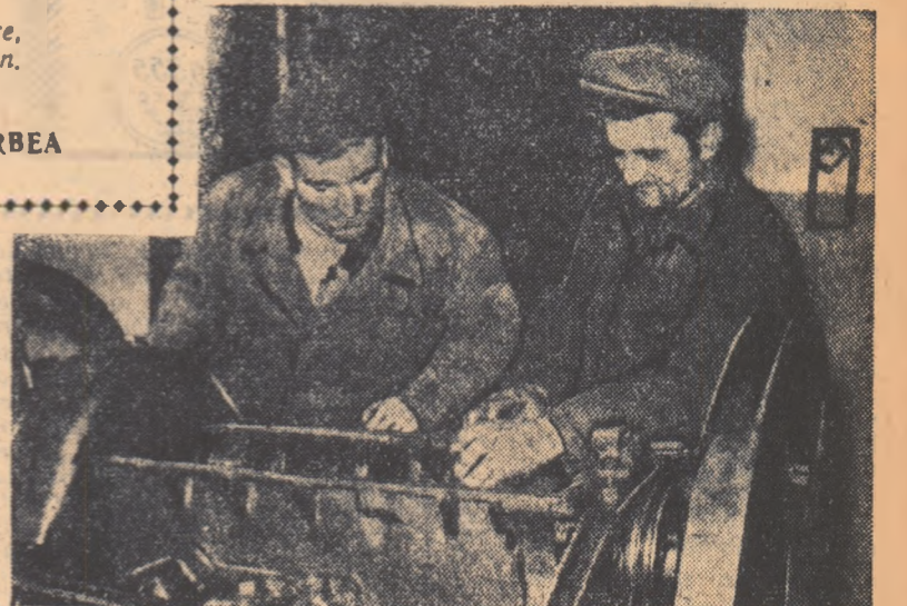
În aceste zile mecanizatorii de la stațiunea de mașini și tractoare Costești, regiunea Pitești, lucrează de zor la reparatul tractoarelor. În fotografie: mecanicul Ion FRĂTESCU și Oprea CIOCAN verifică un vilbrosch de motor K.D.—35. Foto: N. SCARLET
