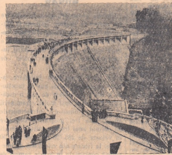
Barajul de la Vir, una din cele mai mari lucrări hidrotehnice construite în ultimii ani de muncitorii și tehnicienii cehoslovaci. Lacul de acumulare al barajului are o capacitate de 56 milioane metri cubi apă. Hidrocentrala de la Vir alimentează cu energie electrică întreaga regiune Cechomoravska Vysocina.
