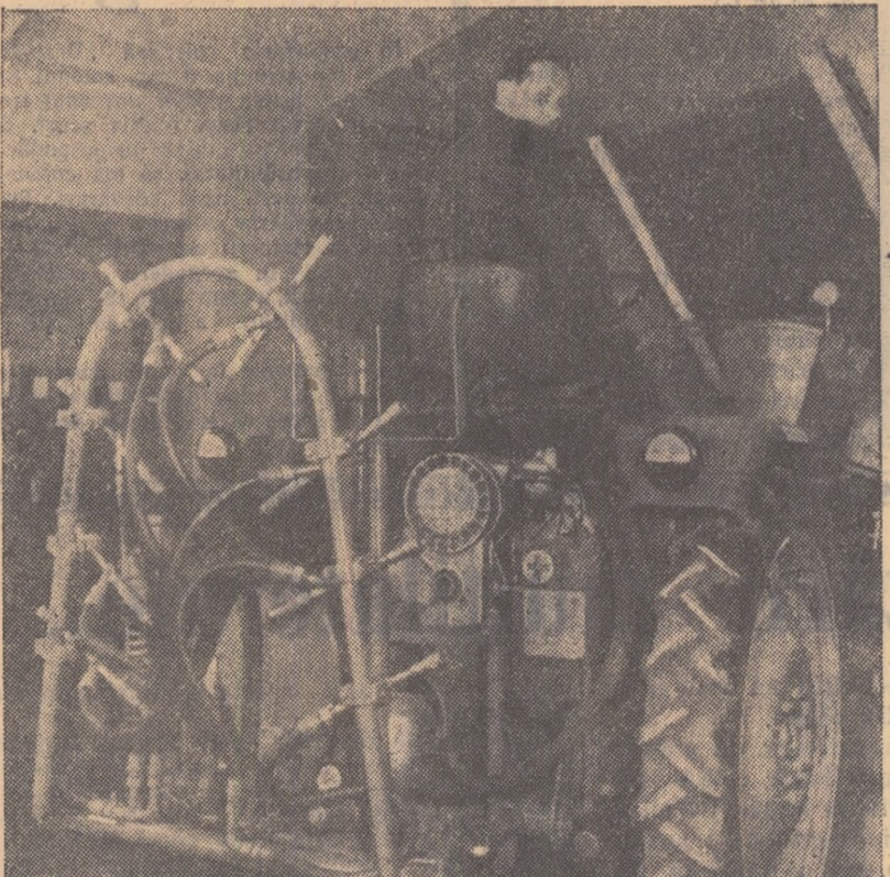
La expoziția permanentă de mostre a R. D. Germană din București a avut loc zilele trecute inaugurarea noii ediții consacrate prezentării unor mașini și aparate pentru combaterea dăunătorilor în agricultură și silvicultură. În fotografie: un agregat pentru combaterea dăunătorilor, purtat de tractor.
