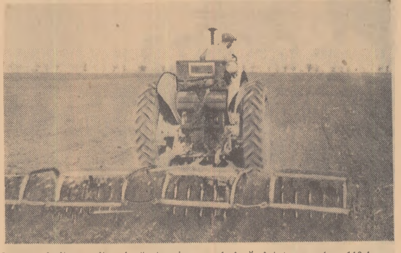
La numai cîteva zile după terminarea de însămînțat a celor 110 ha cu floarea-soarelui, mecanizatorii de la secția Golob a gospodăriei de stat Bulgăruș, raionul Jimbolia, au început prașitul. În fotografie: tractorul Gheorghe Neamtu grăbind cu sapa rotativă locul unde au răsărit deja buruienile. El prașite zilnic cîte 35—38 de ha.
