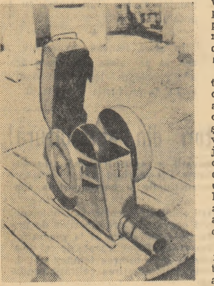
Elevator de apă prin aderență cu capacul deschis
