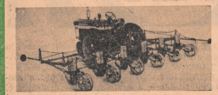
Cele mai diferite specii și varietăți de semințe — începînd cu morcov și terminînd cu mazăre — pot fi semănate cu noul utilaj „Umit 24” fabricat de firma engleză Russels (Kirbymoorside) Ltd. Distanțele reglabile permit semănatul pe 4-5 sau 6 rînduri.
