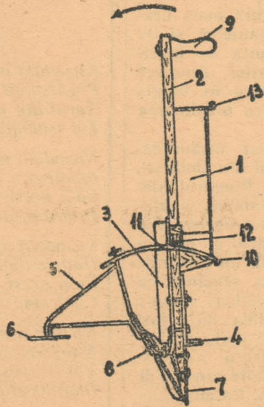
Semănătoarea manuală S.M.—1
