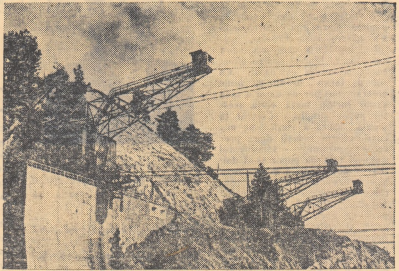
Pe versantul muntelui, se înalță turnurile macaralelor funiculare de la baraj, cu care se transportă benele cu beton.
