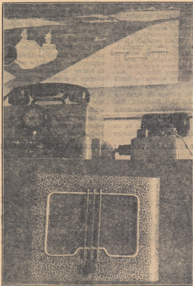
Fotografia reprezintă stația de radio „Urojai” („Recolta”) destinată deservirii colhozurilor, S.M.T.-urilor și sovhozurilor. Cu ajutorul acestei stații se pot face comunicații pe o distanță de 30 km.
