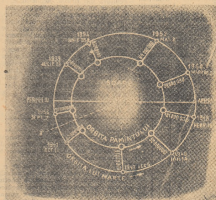
Pozițiile planetei Marte în intervalul 1939—1956. Opozițiile favorabile au loc cînd Marte este aproape de periheliu.
