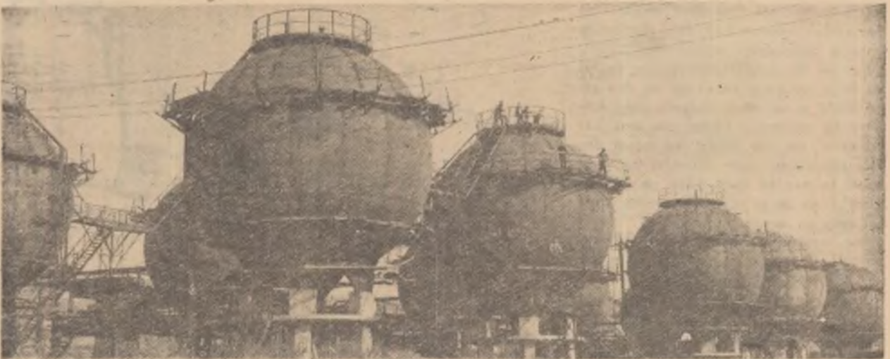
Combinatul de cauciuc Onești. Rezervoarele sferice pentru înmagazinarea butanului, una din materiile prime pentru fabricarea cauciucului. Diametrul unui rezervor este de 10,80 metri, iar volumul de 600 metri cubi.
