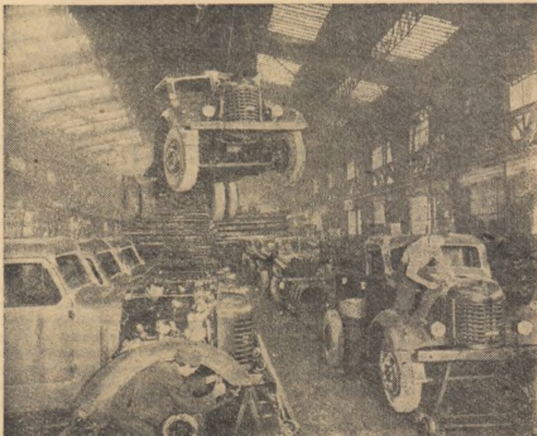
Haia de montaj general a autocamioanelor la uzinele „Steagul Roșu“ din Brașov.
