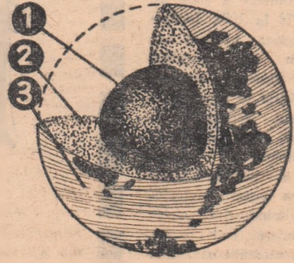
Structura Pământului: 1 — simburele de fier; 2 — zonă bogată în fier și alte metale; 3 — zona exteroară a rocilor pietroase.
