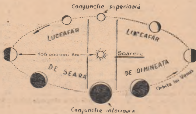
Fig. 1 — Fazele planetei Venus
