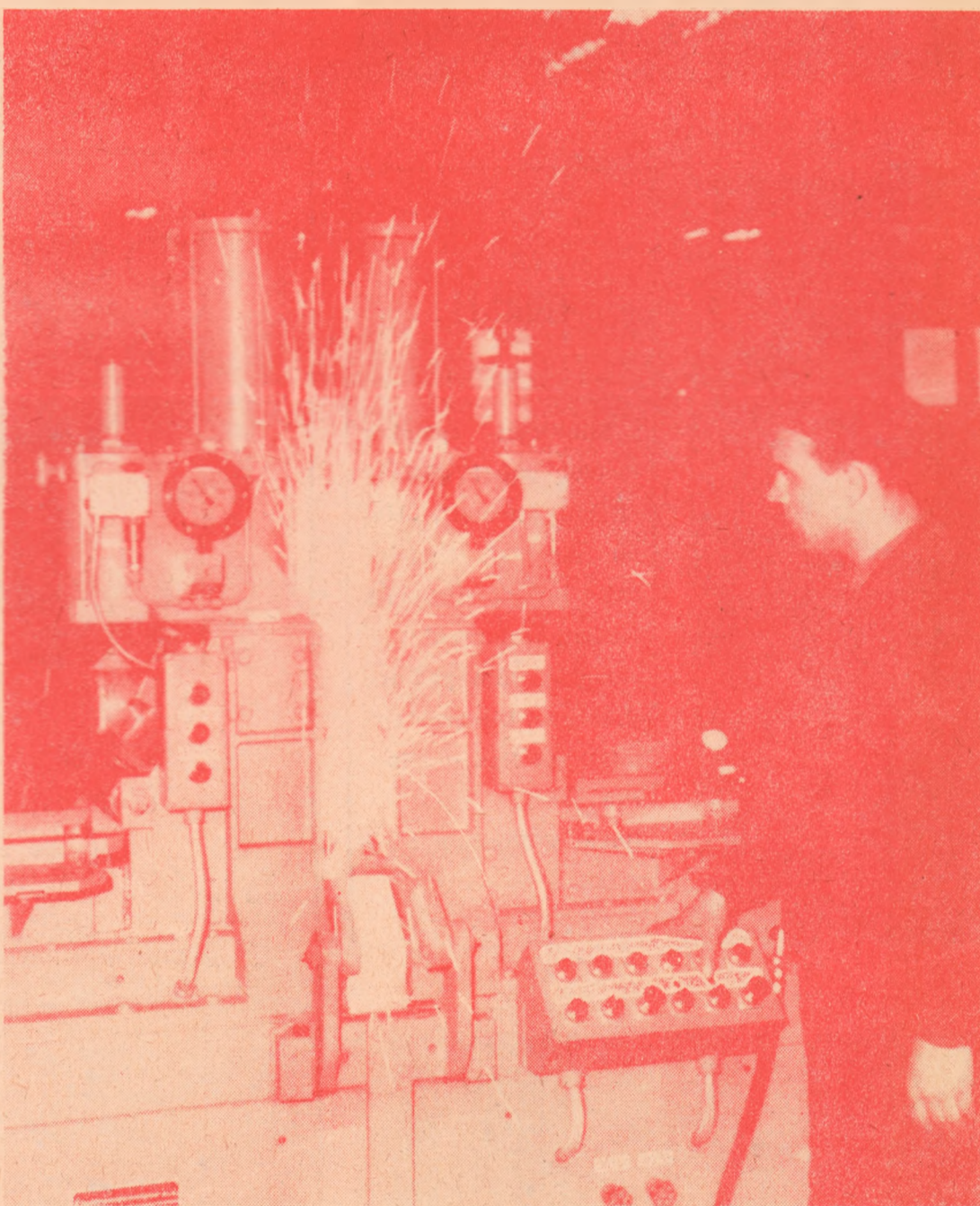
Mașina de sudat ruloirile
