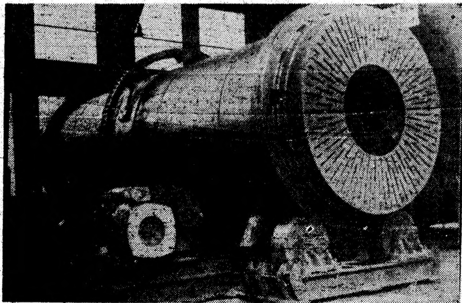
Hidrospălător folosit la preparație.
