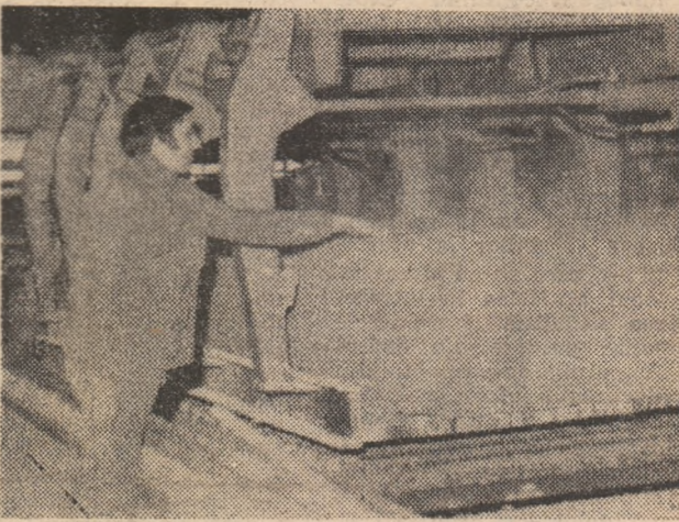
I.M.C. Deva. În foto: Mașina de tăiat beton celular autoclăvizat.
