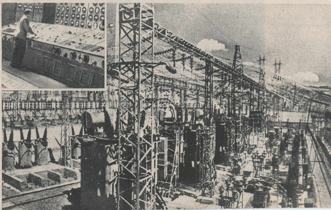
Aspect al hidrocentralei de la Kanaker. În stînga sus: tabloul de comandă.
