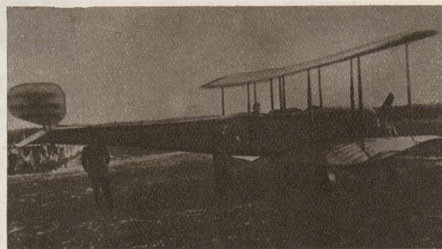
AVIONUL „BRISTOL-COANDĂ”, supranumit „Tractorul”, datorită dimensiunilor lui, excepționale pentru acea vreme. Fotografia a fost făcută la Cotroceni, în 1913. Lîngă avion sînt inginerul H. Coandă, constructorul aparatului, și căpitanul aviator Mircea Zorileanu. În carlingă se află pilotul avionului, căpitanul Andrei Popovici, iar în fața aparatului, mecanicul-aviator Vasile Ionescu.
