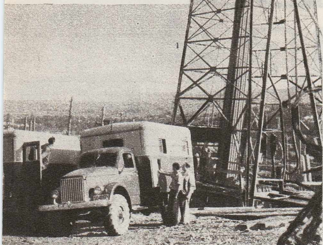
Metoda sovietică de carotaj radioactiv pentru depistarea zăcămintelor de petrol se extinde tot mai mult în industria extractivă petroliferă. În fotografie: camioanele cu instalațiile de carotaj radioactiv au sosit la sonda nr. 2-Băicoi.
