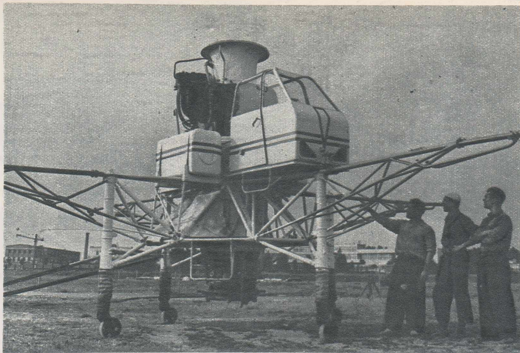
Turboplanul sovietic sau „masa zburătoare”, cum este denumit, constituie un prim pas îndrăzneț, pe calea creării unei aviații care nu are nevoie de aerodroame. Deși aparatul nu are nici aripi, nici elice, el se comportă excelent în aer.
