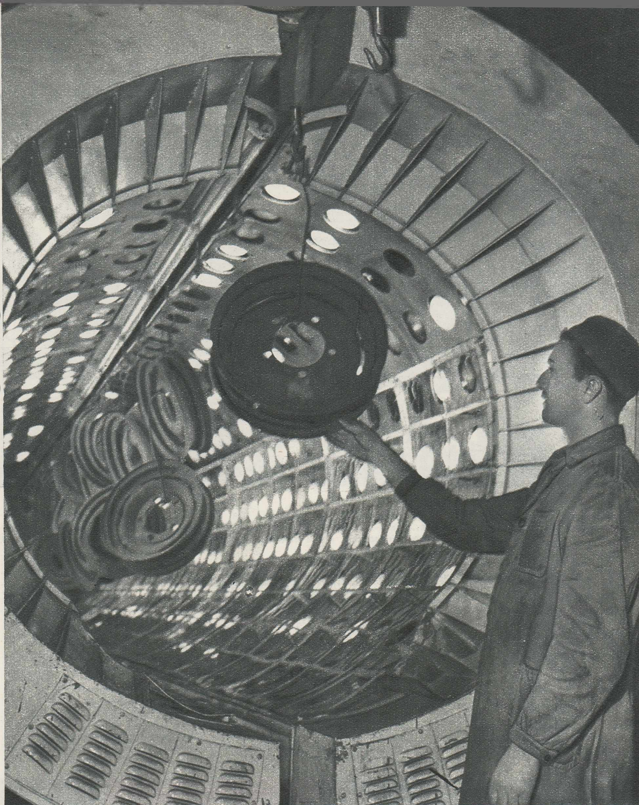
Un tunel cu raze de uscare infraroșii. Prin el trec sute de piese care folosesc la fabricarea tractoarelor.
