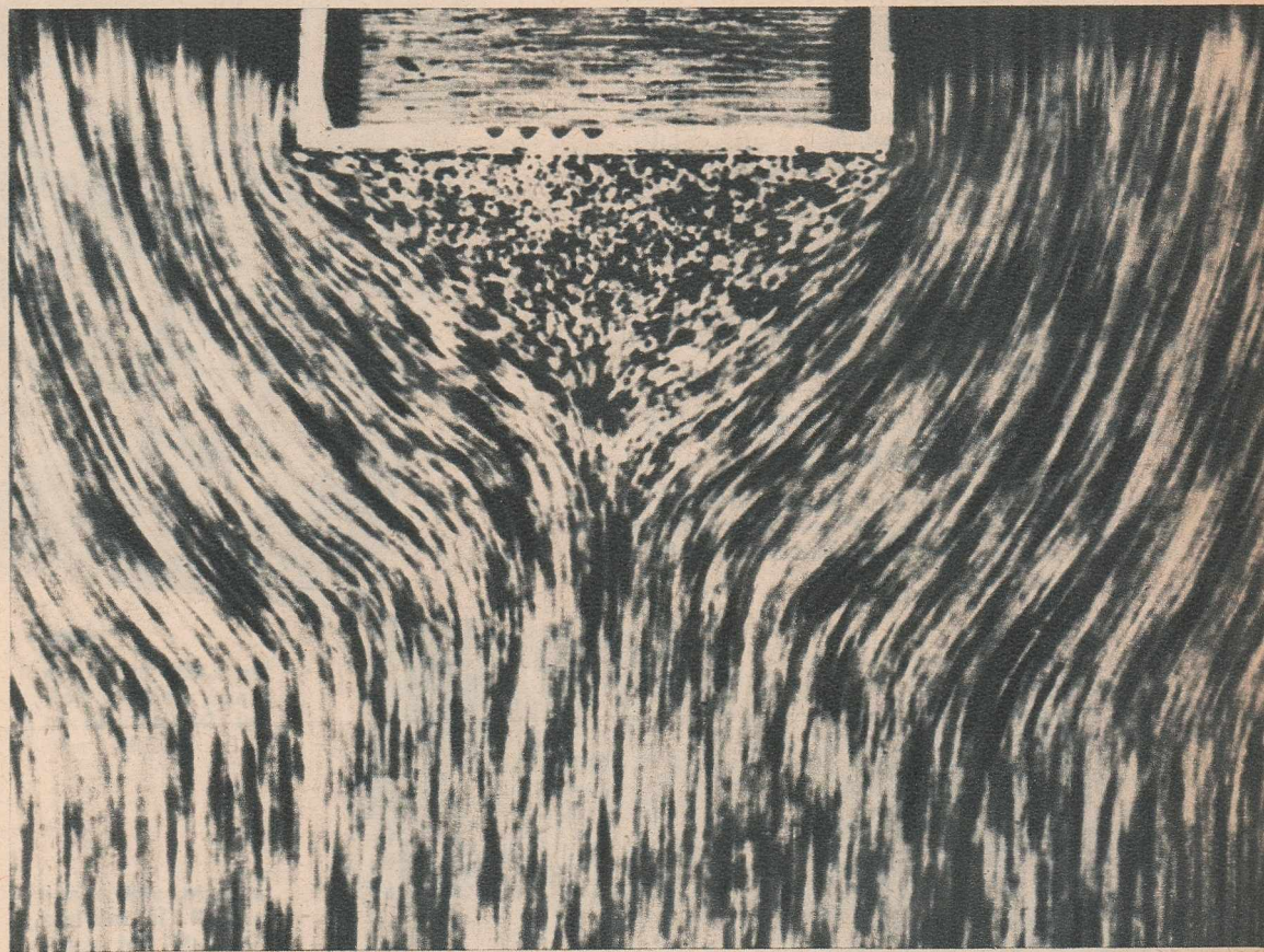
Flăcări? Jocuri de artificii? Nu, ceva mai prozaic, care în termeni științifici se numește „spectrul deformărilor unui masiv de pămînt sub acțiunea unei fundații rigide încărcate”, iar în vorbirea curentă, studiul deplasării particulelor de pămînt sub o fundație.
