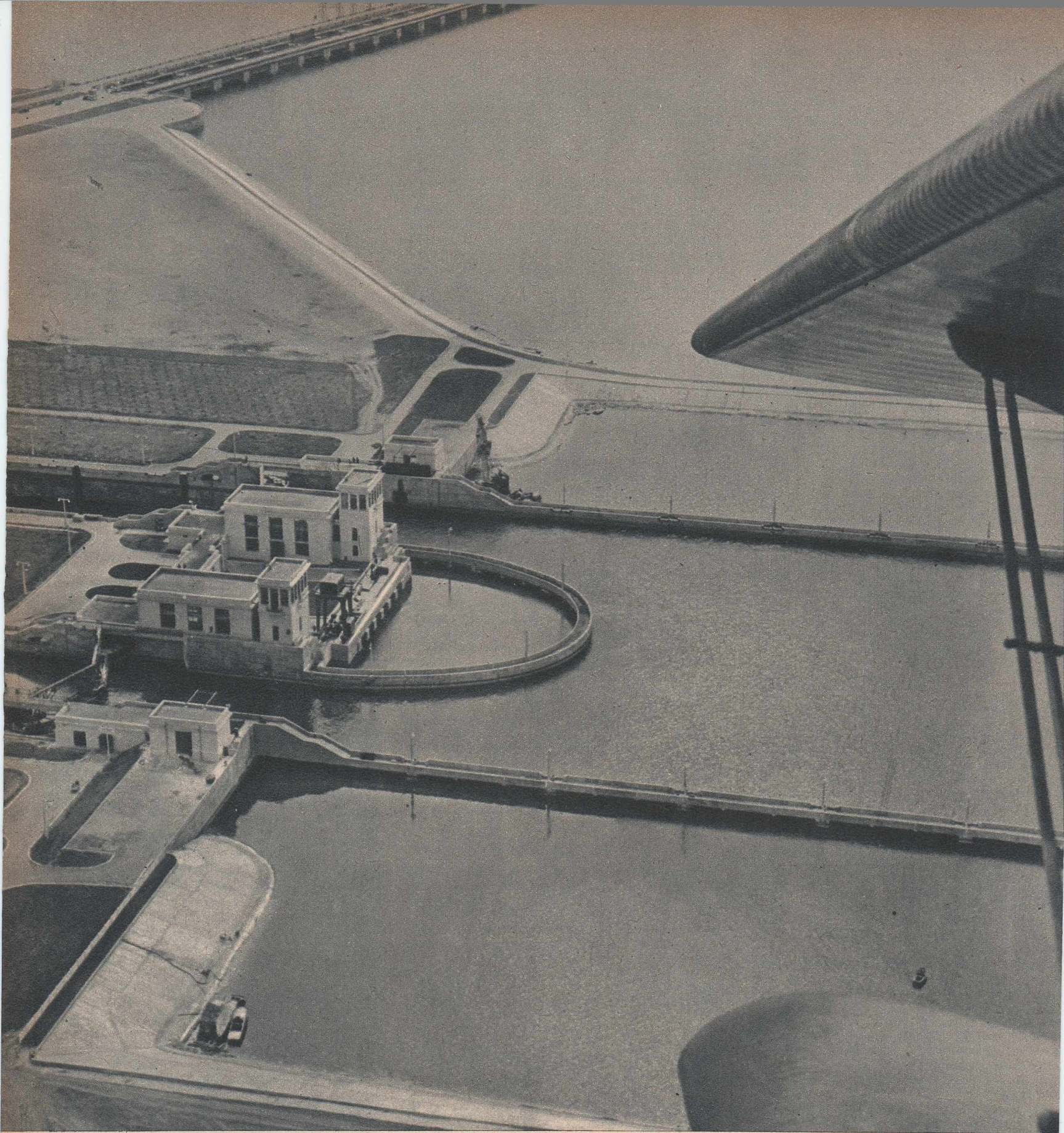
Hidrocentrala „V.I. Lenin” văzută din avion.
