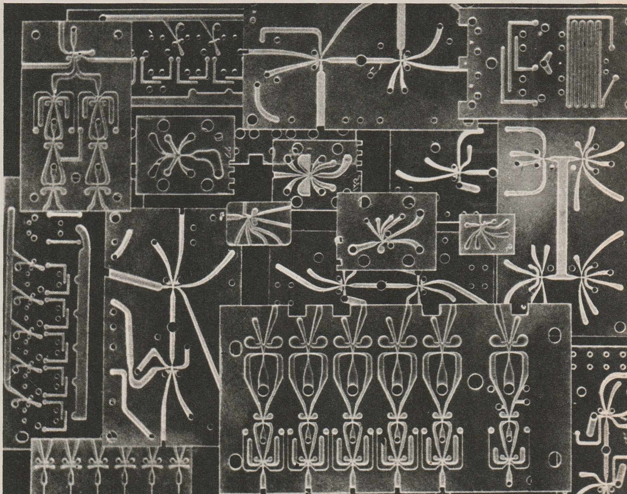
Această imagine nu reproduce un panou decorativ oarecare (cum s-ar putea crede), ci o parte din circuitele unei instalații de transmitere a datelor asupra producției într-o uzină, instalație bazată pe principiul transmiterii de fluide în circuite închise.
