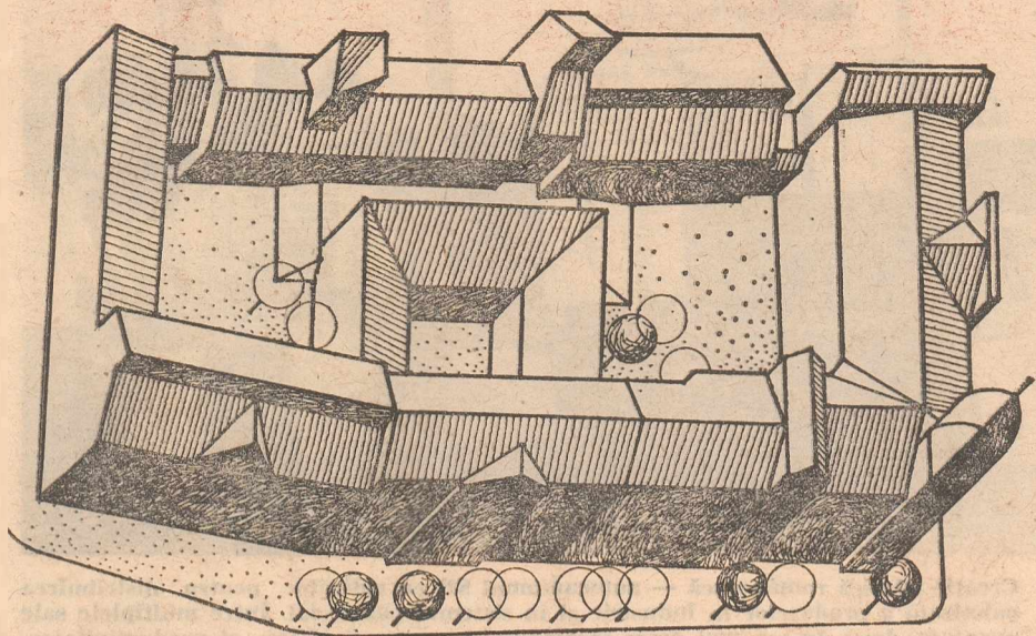
Latura de sud a Pieței Libertății. Propunere de organizare a zonei culturale dintre Muzeul de istorie și Biblioteca județeană, după proiectul studenților. Se pot observa, în desen, extinderile în curte, supraetajările și refacerea volumelor inițiale
