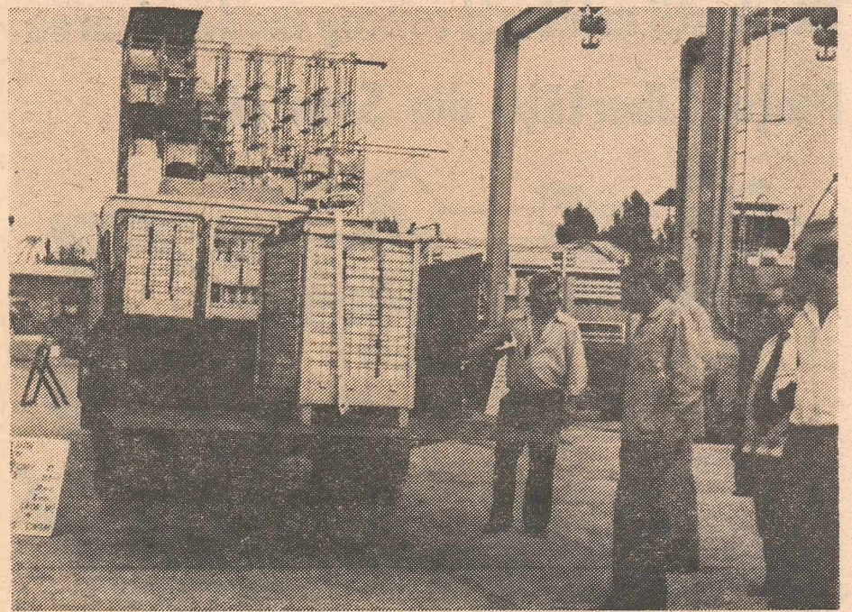
Creare tehnică românească — autocamionul SR cu ridicător pentru distribuirea palelizată a produselor în industrie și în sistemul comercial. Intre multiplele sale avantaje, două de cea mai mare însemnătate: operativitatea și productivitatea. Fotografie de EMANUEL TANJALA
