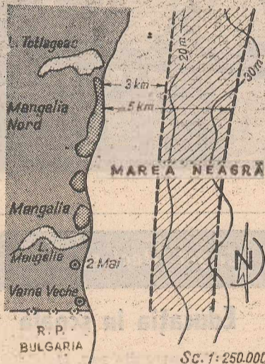
Zonă favorabilă amplasării stației pilot pentru captarea energiei valurilor.
