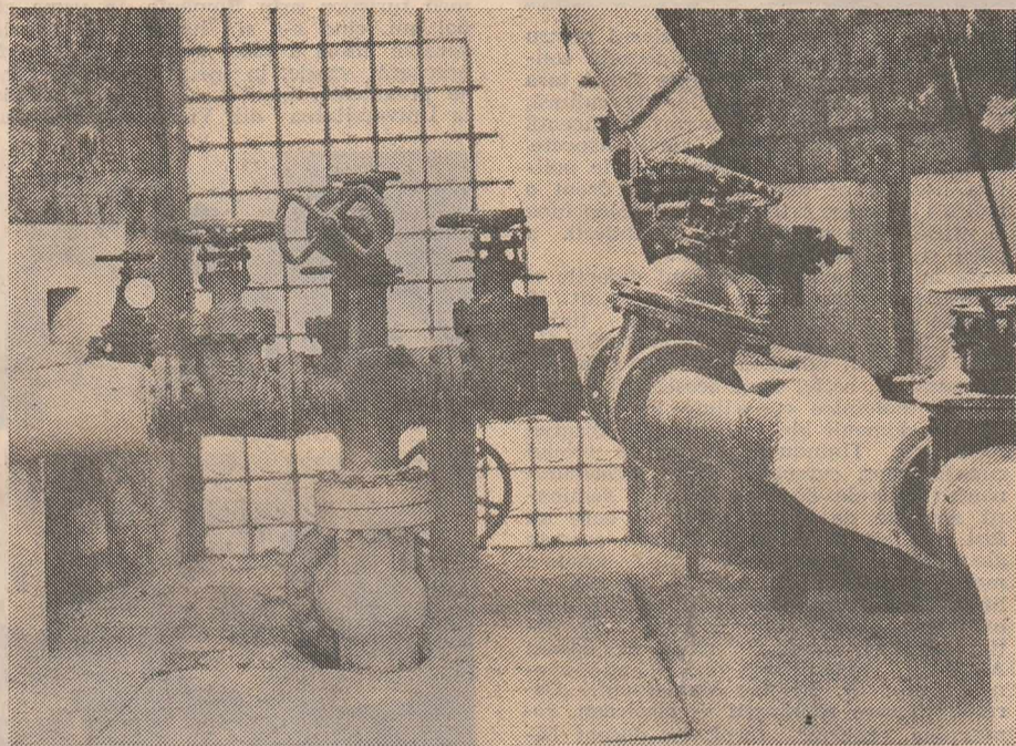
Acest cap de foraj cu racordurile de distribuție, aparținînd sondei cu numărul 4005 din Oradea, asigură, încă de acum 8 ani, cu bune rezultate, încălzirea centrală a 12 apartamente, încălzirea unui dispensar, a unui restaurant și a unei expoziții permanente de plante exotice. Temperatura apei, 80 de grade; debitul sondei, 12 litri pe secundă.
