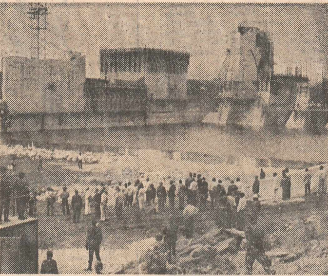
Faza finală de execuție a digului sistemului de hidroameliorare de pe riul Umbeluzi, în localitatea Pequenos Libombas din provincia Maputo. (R. P. Mozambic).
