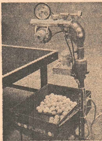
Magazia de mingi și „tunul” robotului, capabil să imprime mingii direcția și viteza dorite.
