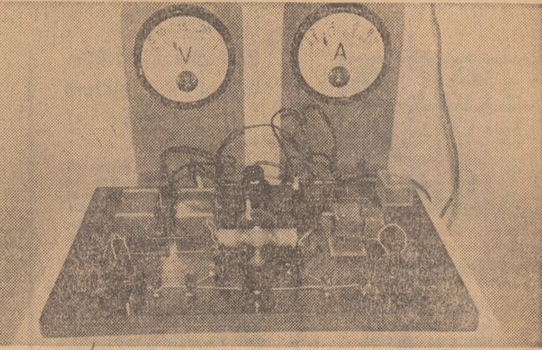
Aparat pentru verificarea legii lui Ohm în curentul alternativ, construit la Liceul nr. 15 din București
