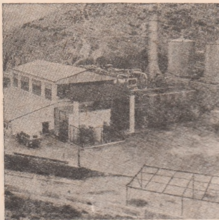
Uzină de desalinizare a apei de mare, cu o capacitate de 400 t apă potabilă, în insula Ceuta
