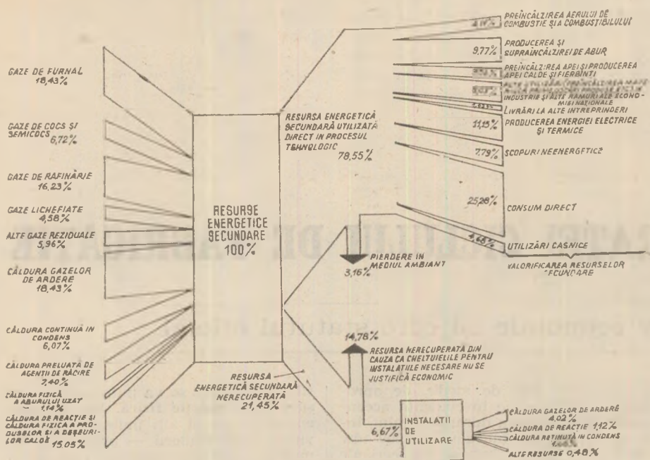
Fig. nr. 4. Utilizarea resurselor energetice secundare
