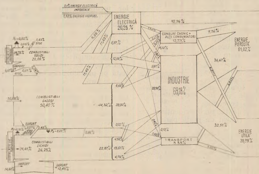
Fig. nr. 1. Fluxul energetic în 1976 în R.S. România
