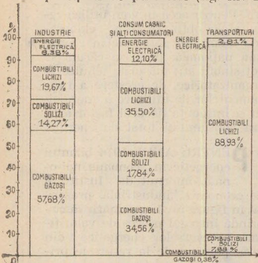
Fig. nr. 2 Utilizarea energiei în 1976 pe tipuri de purtători de energie
