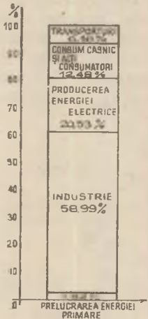
Fig. nr. 3. Pierderi totale de energie
