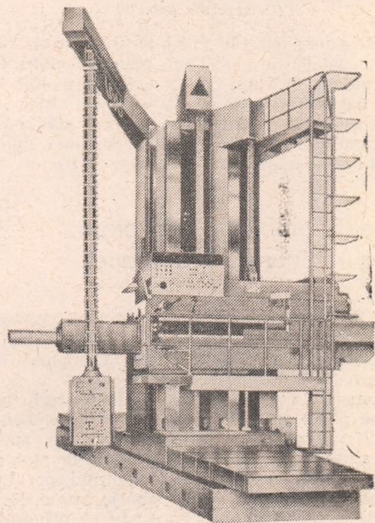
Printre cele mai noi tipuri de mașini-unelte de mare productivitate și precizie figurează și mașina orizontală de alezat și frezat cu pinolă AFP 130A. Recenta realizare a întreprinderii de mașini-unelte și agregate din București este cea mai mare și cea mai grea mașină-unelte fabricată vreodată în România: măsoara 16 000 mm lungime, 4 000 mm lățime, 8 000 mm înălțime și cîntărește nu mai puțin de 130 000 kg! Comanda ușoară a mașinii-gigant este asigurată prin concentrarea comenzilor principale pe un tablou mobil suspendat și pe un panou de comandă fix. Această mașină realizată în concordanță cu cele mai severe exigențe ale tehnicii actuale are termen de garanție 15 ani de zile.
