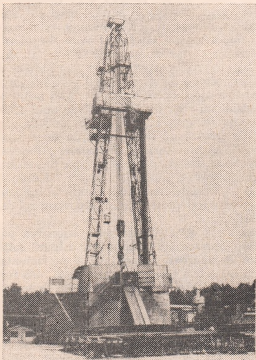
Seria instalațiilor de foraj, în a căror execuție întreprinderea ploieșteană „1 Mai“ ocupă în ultimele două decenii un loc de primă mărime pe plan internațional, a fost completată în anii acestui cincinal cu un prestigios produs: instalația de foraj F-500 DEWL capabilă să forceze sonde pînă la adîncimi de 10 000 metri. Dintre performanțele acestei instalații, una dintre cele mai puternice și mai moderne realizată pînă acum pe plan mondial, semnificative sînt: sarcina maximă de lucru la cîrlig — 500 tf; puterea totală instalată — 7 500 C.P.; puterea maximă de antrenare a trolului — 3 000 C.P.; numărul vitezelor la masa rotativă: 2+2R. Concepția acestei noi instalații se remarcă prin simplificarea la maximum a lucrărilor de montaj, cit și a celor impuse de pregătirea terenului în care lucrează.
