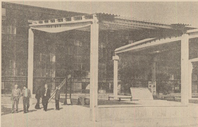
Fotografia prezintă, din expoziție, o secțiune exemplificativă de hală neincalzită pentru procese tehnologice calde, depozite și magazii, avînd distanța între stâlpi de 12—15—18x6 m, acoperișul din pane pe grinzi cu înălțime variabilă și cu goluri, luminatorul (în planul învelitorii) din plăci ondulate din mase plastice și învelitoarea din azbociment ondulat. Indici pe mp: greutate proprie 150 kg, consum de oțel 8,5 kg, consum de ciment 35 kg, manoperă de montaj 1,2 ore-om.
