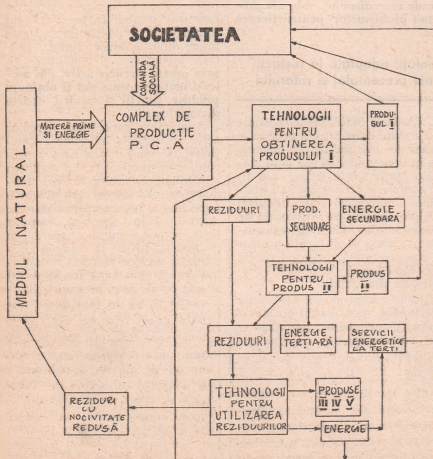
Schema circuitului materiei și energiei într-un complex de producție bazat pe procesul circular activ
