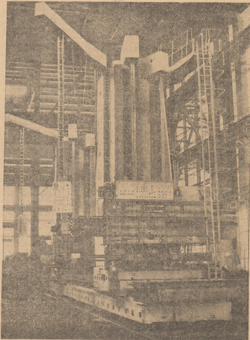
Mașina orizontală de alezat și frezat tip AFB—180
