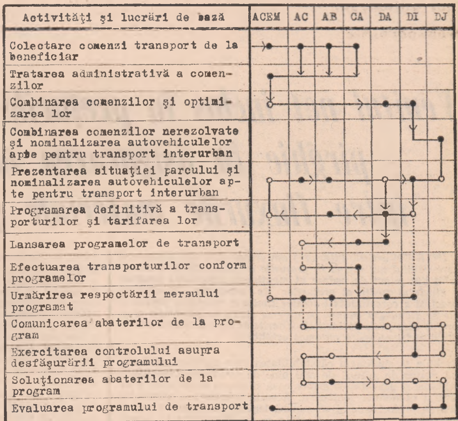
Fig. 2 : Diagrama de rutină a conducerii transporturilor auto prin dispeccer. ACEM — agenția de colectare și expediere mărfuri ; AC — autocoloană ; AB — autobază ; CA — conducător auto ; DA — dispeccer autobază ; DI — dispeccer interurban I.T.A. ; DJ — dispeccerat județean
