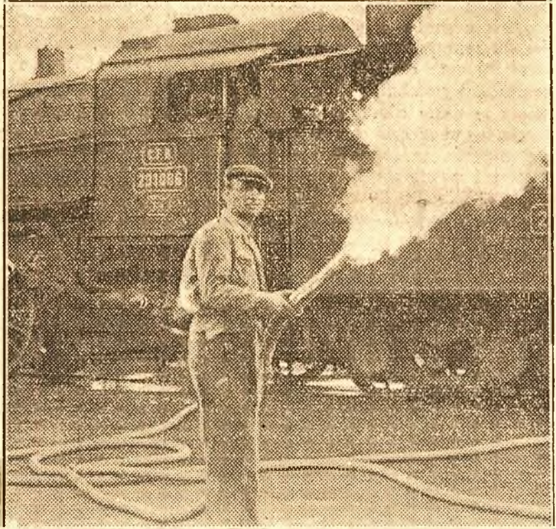
Tovarășul Tane Gheorghe, muncitor la depoul B.C. Grivița, manipulează aparatul pentru desinfecțarea cu aburi, supraîncălzit a magaziiilor de cereale. Aparatul este pus în legătură cu cazanul locomotivei.
