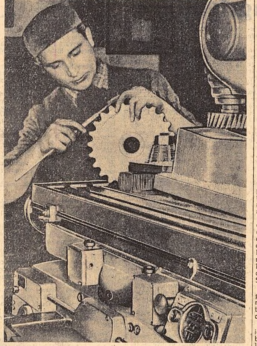
Frezorul Marin Burdulea din secția a VI-a a atelierelor de uzină „Semărădăra” din Capâlnă este cunoscut în întreprinderea în care lucrează ca un muncitor cu o bună pregătire profesională, care folosește din plin tehnica nouă. Lucrînd la o freză universală el reușește, printre alii, să organizeze o lucră de muncă și prin folosirea unor metode înaintate, să-și depășească în medie sarcinile de plan cu circa 150%. In clișeu: Frezorul Marin Burdulea la locul său de muncă.
