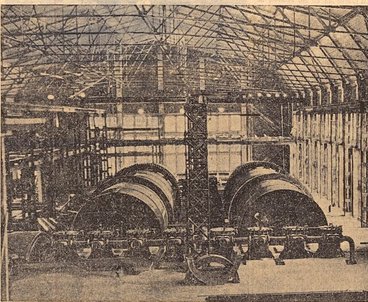
La Livezi, regiunea Craiova, se desfășoară din plin lucrările de construcție a unei noi și moderne fabrici de zahăr. Înzestrată cu utilaje perfecționate, de mare randament, noua fabrică va avea o mare capacitate de producție. În prezent se lucrează la montarea instalațiilor și agregatelor care vor intra în probă la sfîrșitul acestui an.
