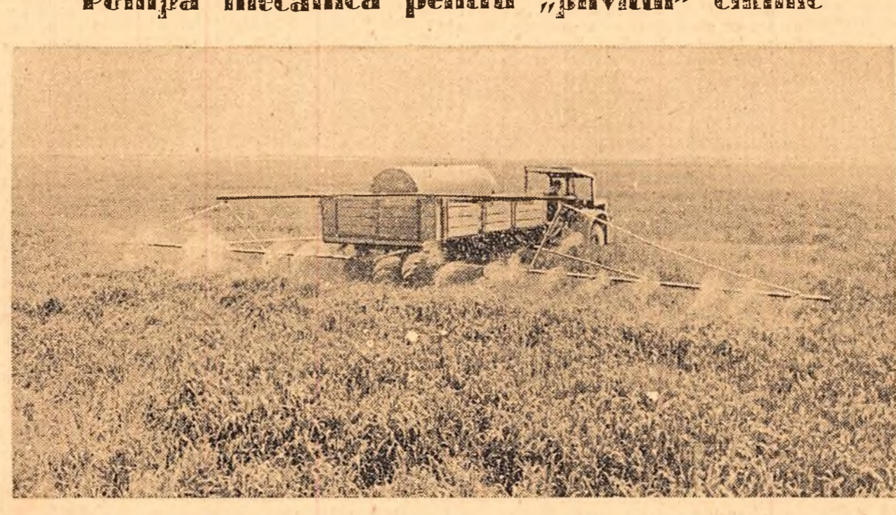
Cercetînd pompa sovietică OKS, un colectiv de ingineri și tehnicieni de la gospodăria de stat Moșneni (Constanța) a construit din resurse locale o pompă mecanică pentru stropirea culturilor cu ierbicidul 2-4 D care distruge buruienile. Cu ajutorul acestei pompe se pot stropi zilnic 70 ha. În clișeu: Pompa mecanică pentru „plivitul” chimic, realizată la G.A.S. Moșneni.
