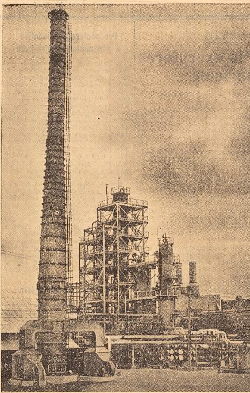
La rafinaria nr. 10 Borzești se execută ultimele lucrări pentru darea în producție a primei instalații de cracare termică. Utilajele — de cea mai înaltă tehnică — sînt construite în Uniunea Sovietică. Instalația de cracare termică va produce benzina auto și va folosi ca materie primă păcura provenită de la instalația de distilație atmosferică și vid, care pînă acum se întrebuința drept combustibil. Acum, în întrecerea saștilor în cinstea zilei de 1 Mai, constructorii și montatorii de pe șantier muncesc intens pentru a pune în funcțiune înainte de termen noua instalație.
