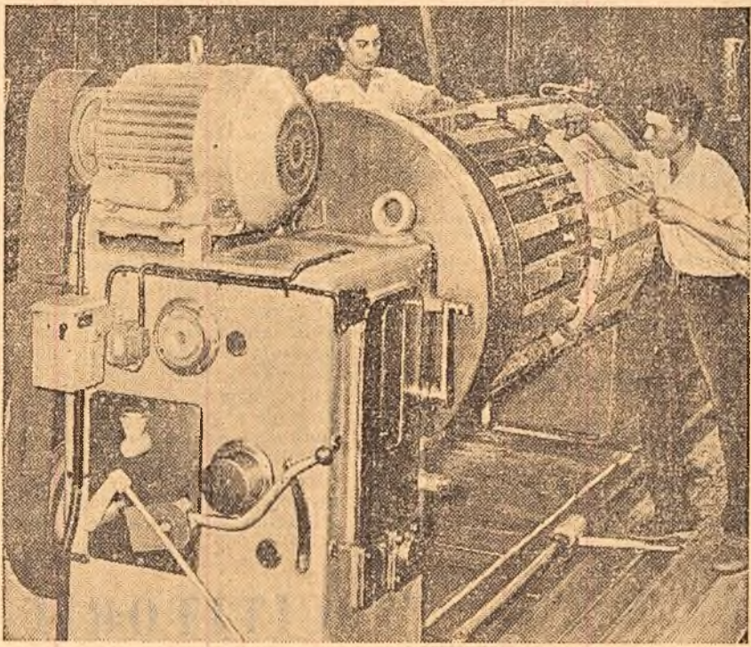
În atelierul de bobinaj al sectorului de transformatori al fabricii „Electro-Putere din Craiova — atelier dotat cu numeroase mașini moderne — se execută, printre altele, și bobine pentru transformatori de puteri mari. În clișeu: Bobinatorii Bancu Ștefan și Popescu Margareta lucrînd la confecționarea unei bobine. (Foto: G.H. VINTILA)
