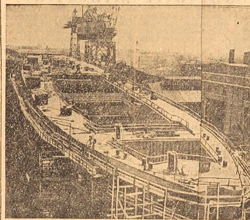
La șantierul naval din Leningrad, înaintea cu reziznice lucrările de construcție a spărgătorului de gheață „Lenin” — primul spărgător de gheață din lume înzestrat cu un motor atomic.
