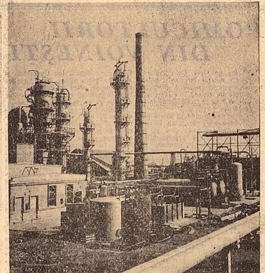
Noua instalație de distilare atmosferică vacuum, de la rafinăria din Onești, intrată nu de mult în funcțiune.
