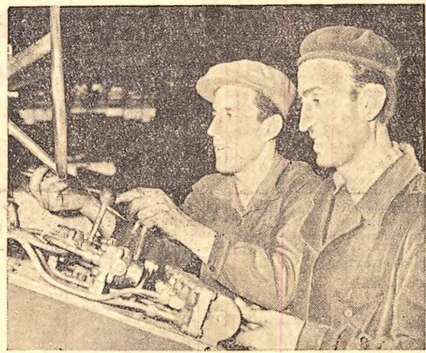
Colectivul uzinelor „1 Mai”-Ploesti a dobândit o experiență valoroasă în ce privește fabricarea utilajului petrolifer. O instalație modernă de foraj este montată aici în numai șase zile. În fotografia de față, pe montorii Gh. Drăgan și Const. Bulac lucrând la montarea pupitului de comandă al unui troliu. (Foto Gh. Vințilă)
